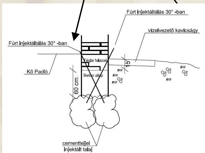
Keresztmetszet
